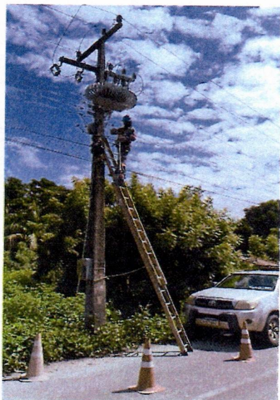
Figura 06: equipe em campo realizando substituições necessárias de Lâmpadas, cabo elétrico, conector, reator, arruela, braços com caminhonete adaptada.
