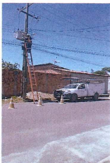
Figura 02: equipe em campo realizando substituições necessárias de Lâmpadas, cabo elétrico, conector, reator, arruela, braços com caminhonete adaptada.
