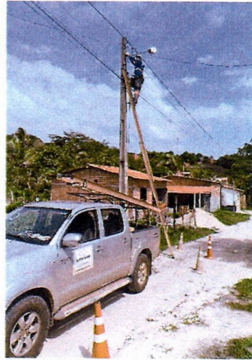
Figura 03: equipe em campo realizando substituições necessárias de Lâmpadas, cabo elétrico, conector, reator, arruela, braços com caminhonete adaptada.
