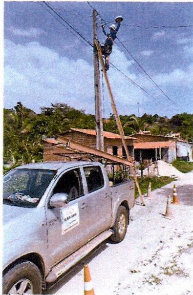
Figura 04: equipe em campo realizando substituições necessárias de Lâmpadas, cabo elétrico, conector, reator, arruela, braços com caminhonete adaptada.
