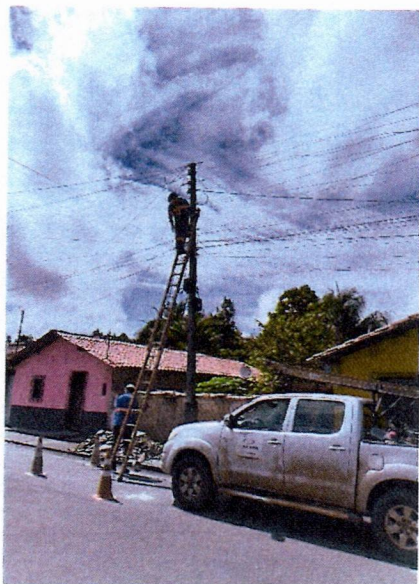
Figura 05: equipe em campo realizando substituições necessárias de Lâmpadas, cabo elétrico, conector, reator, arruela, braços com caminhonete adaptada.
