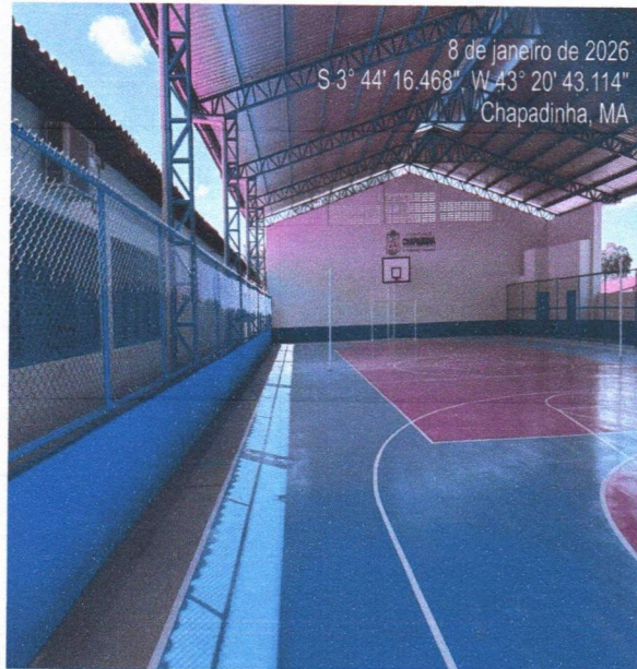
IMAGEM 3: execução de alambrado, mureta, , piso da quadra com marcação
