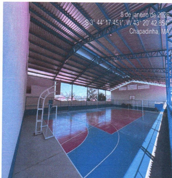
IMAGEM 6: execução de cobertura metálica, iluminação com refletores, piso da quadra e equipamentos
