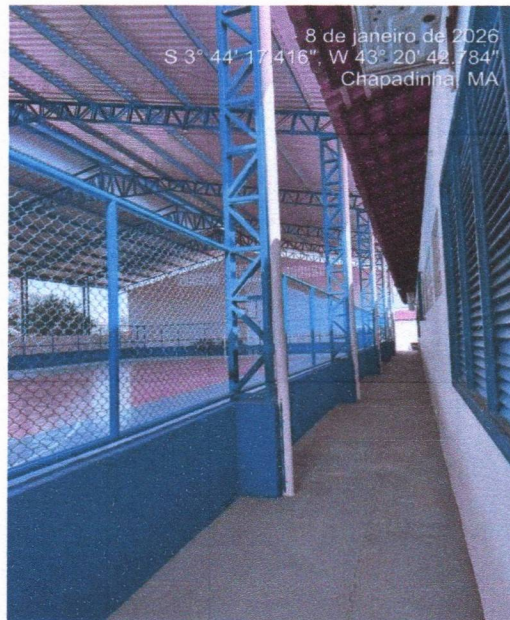
IMAGEM 7 execução de alambrado e drenagem de águas pluviais
