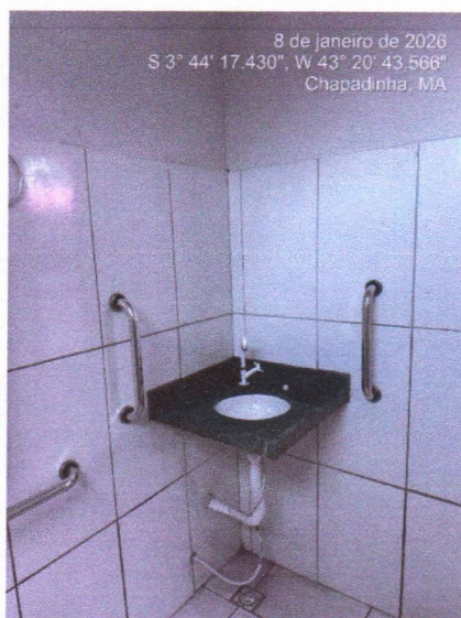
IMAGEM 14: execução do banheiro PCD, incluso vaso sanitário, lavatório e barras de apoio
