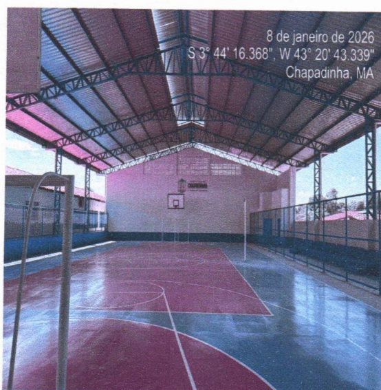
IMAGEM 2: cobertura metálica, piso da quadra e equipamentos
