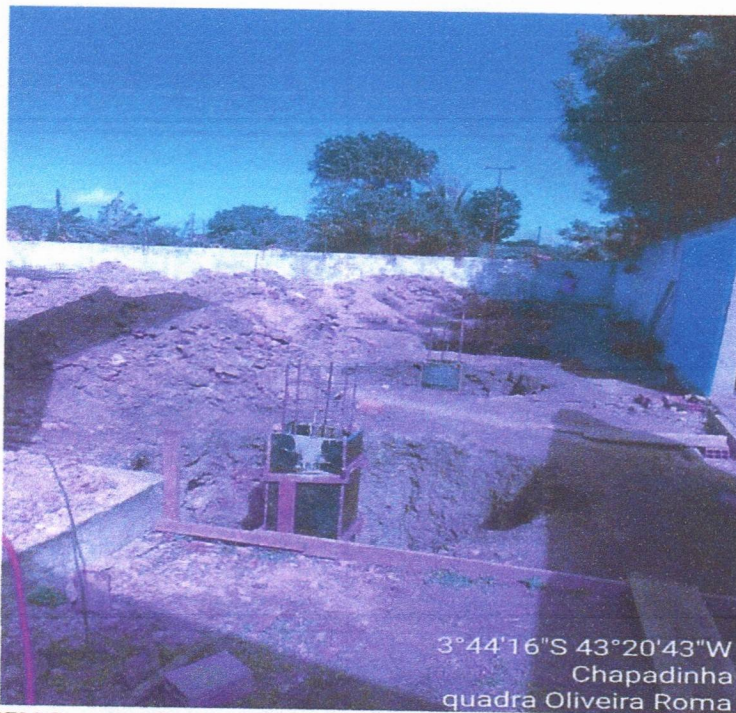
IMAGEM 8: execução das fundações – sapatas isoladas de concreto armado
