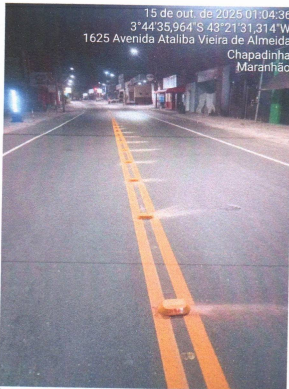
Imagem 03 – SERVIÇOS DE PINTURA E TACHÕES
