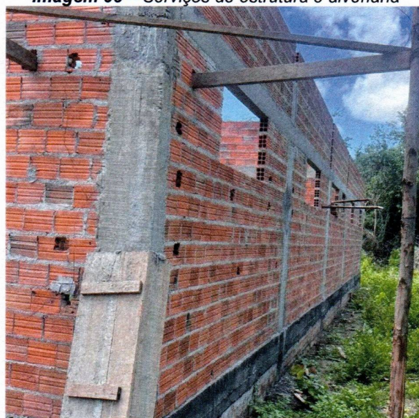
Imagem 09 – Serviços de estrutura e alvenaria..
