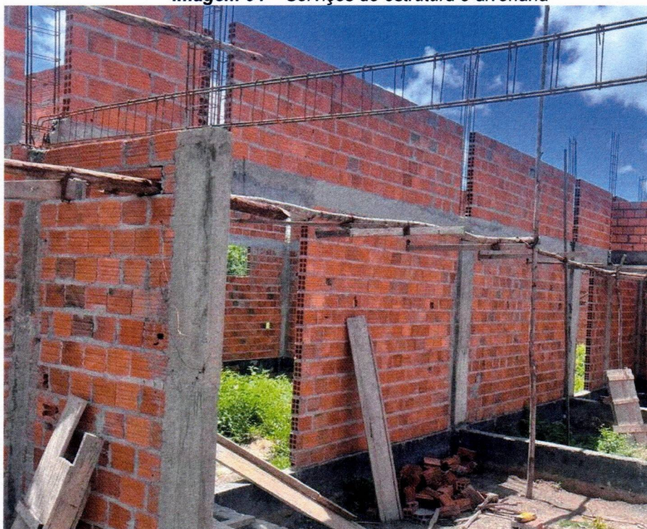
Imagem 05 – Serviços de estrutura e alvenaria
