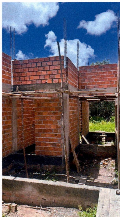
Imagem 6 – Execução da alvenaria, concretagem dos pilares e armação das vigas superiores.
