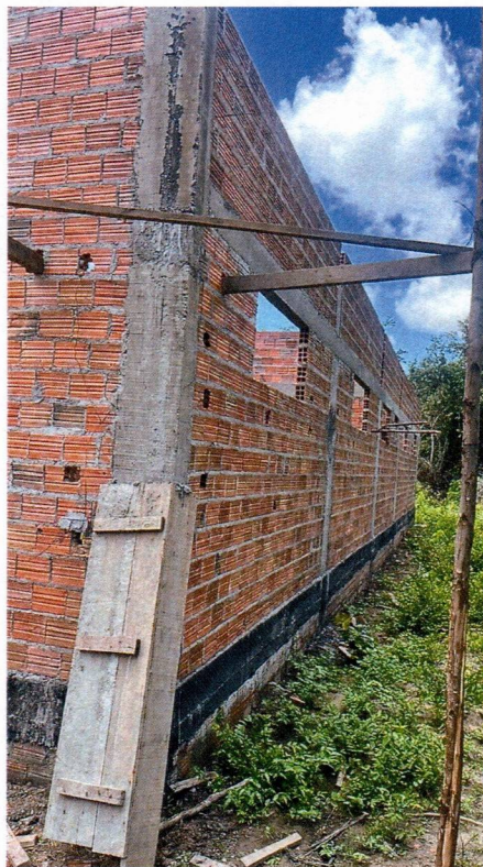
Imagem 4 – Execução da alvenaria, concretagem dos pilares e armação das vigas superiores.
