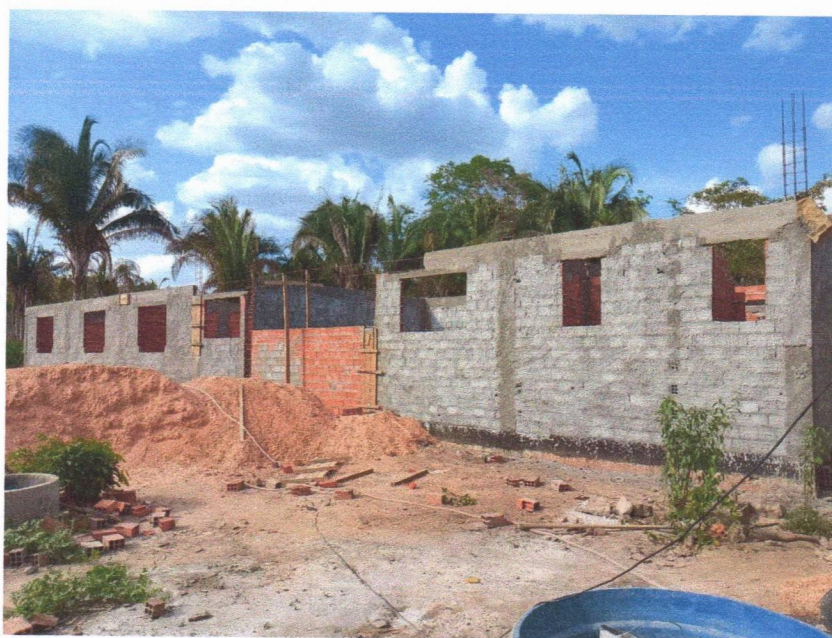
Imagem 6 – Execução da viga superior e do chapisco.
