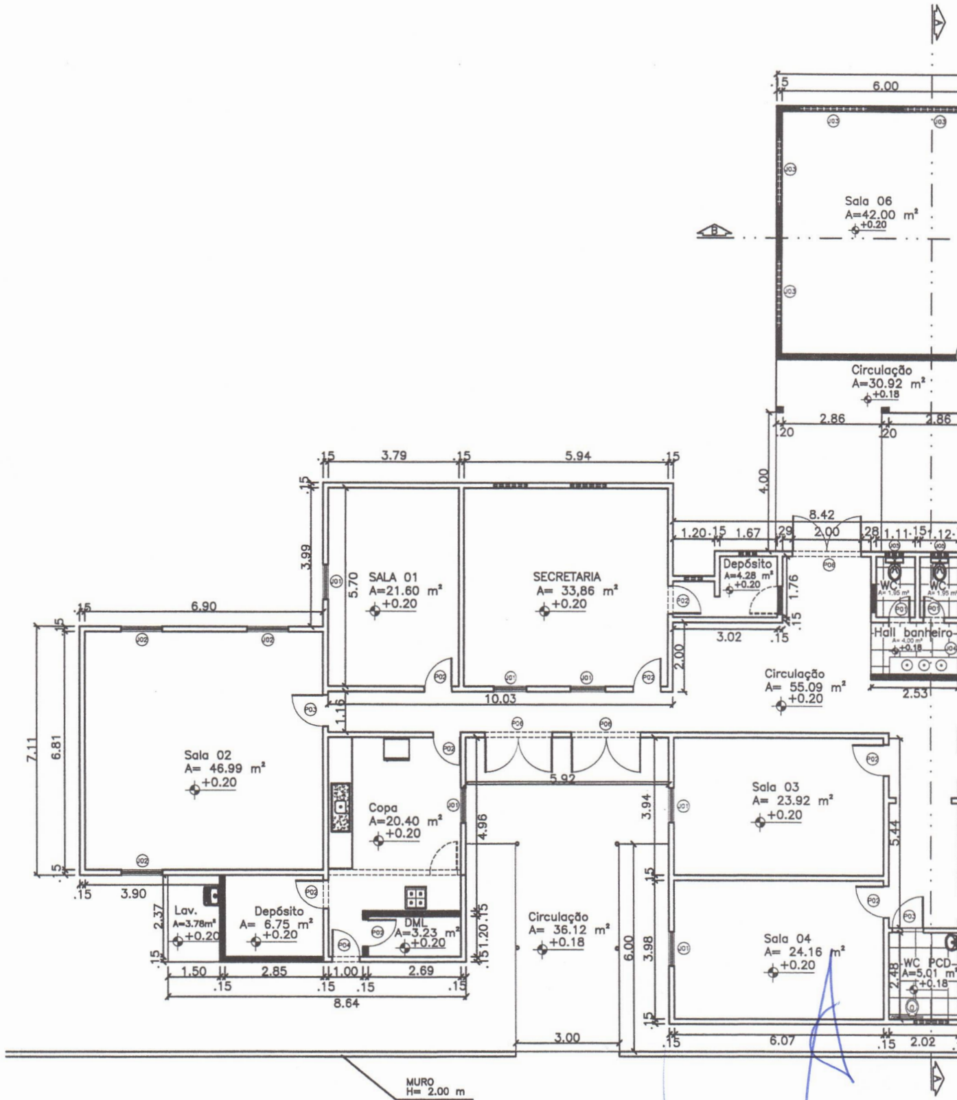
PLANTA REFORMA esc 1:150
