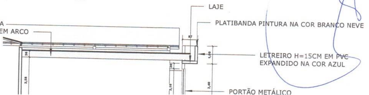
2 FACHADA PRINCIPAL (SUL) ESCALA 1 : 125
