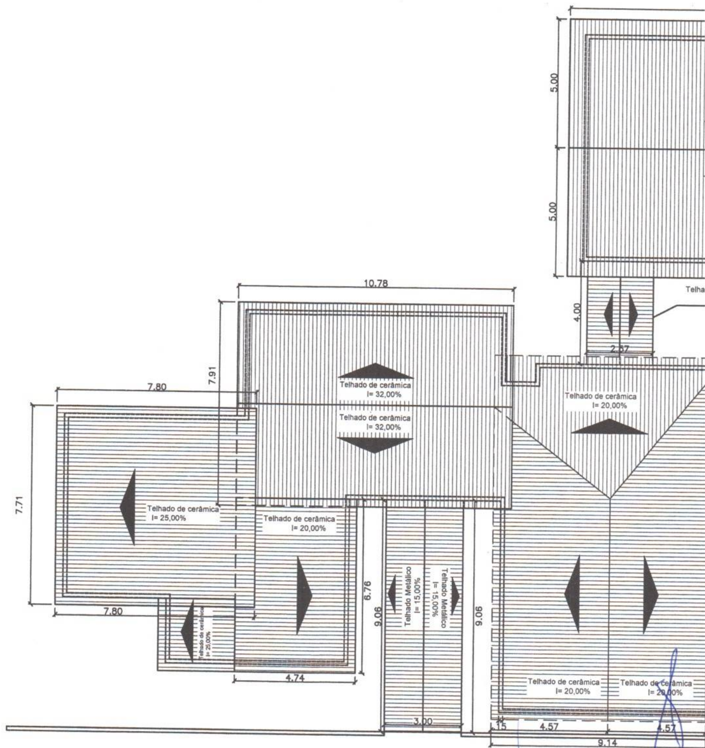
PLANTA DE COBERTURA esc 1:150
