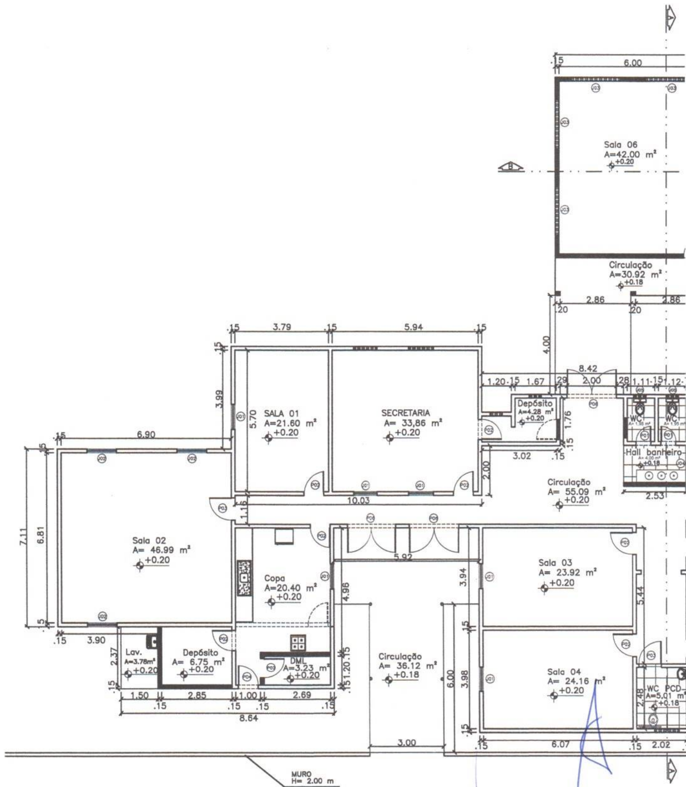
PLANTA REFORMA esc 1:150
