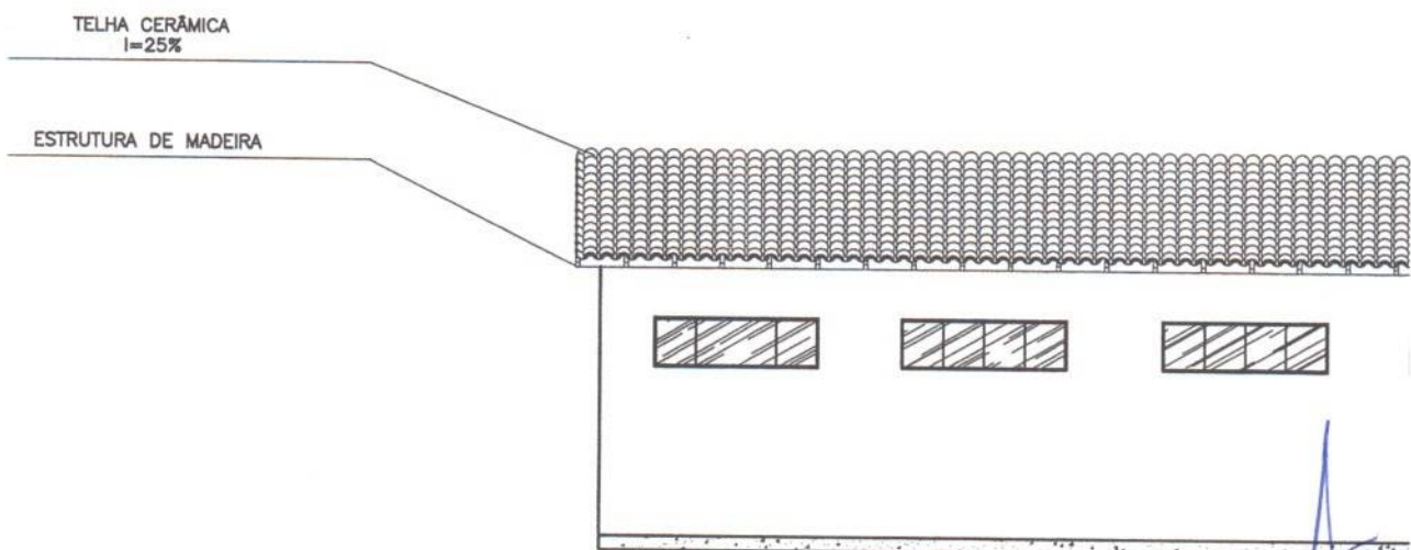
FACHADA SUL esc 1:100
