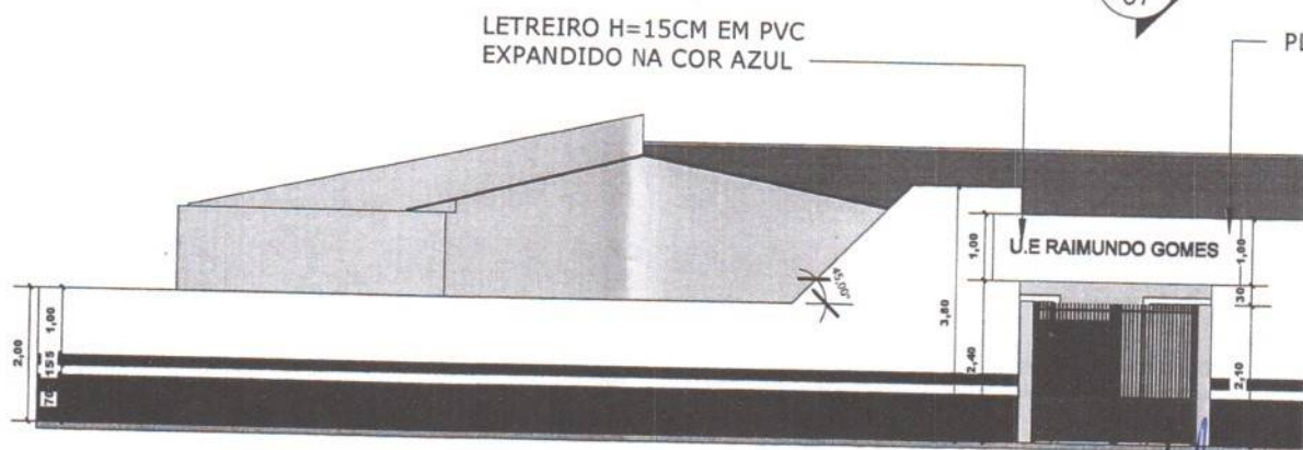
2 FACHADA PRINCIPAL (SUL) ESCALA 1 : 125
