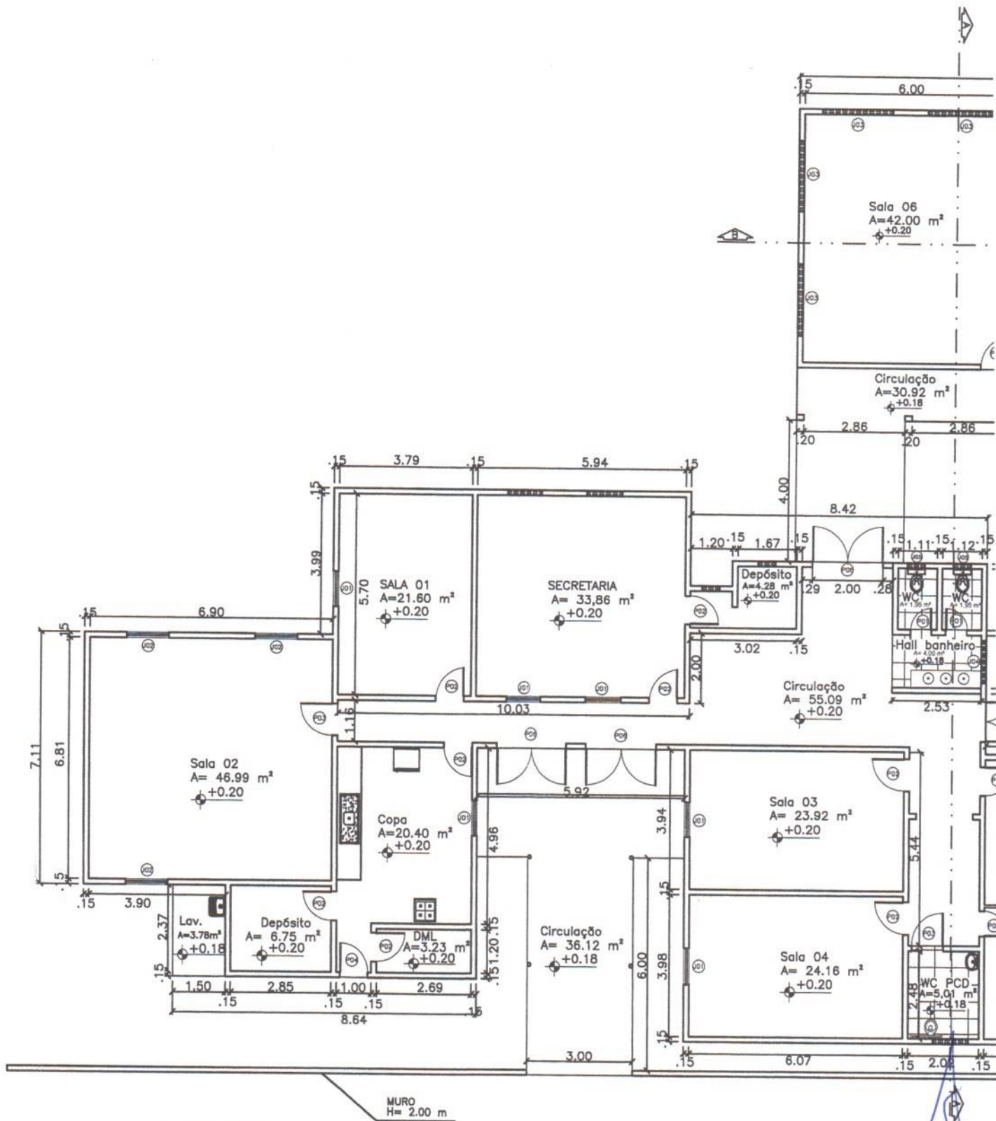
PLANTA BAIXA esc 1:150
